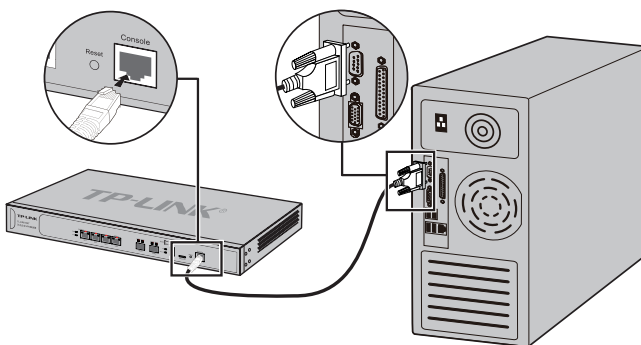
图3-3 Console端口连接示意图
